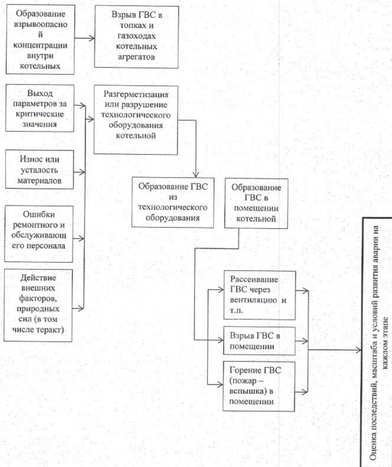
Рисунок 2. Схема построения сценариев развития аварий в замкнутом объёме (в помещении или в котле) с указанием основных причин их возникновения
