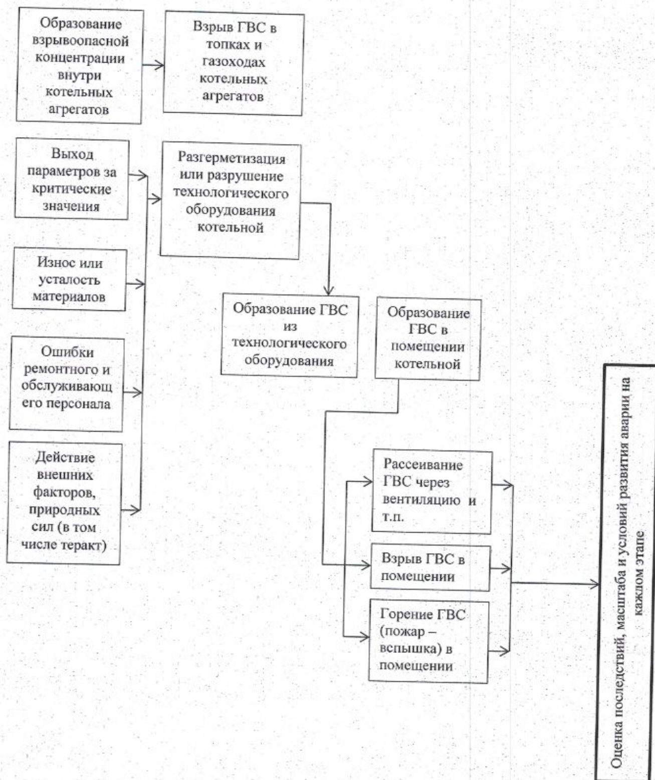
Рисунок 2. Схема построения сценариев развития аварий в замкнутом объеме (в помещении или в котле) с указанием основных причин их возникновения
